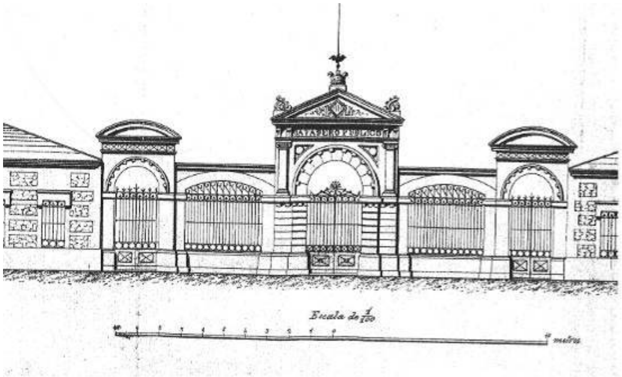
Alzado de la fachada principal. © Archivo Histórico de la Ciudad de Valencia.
