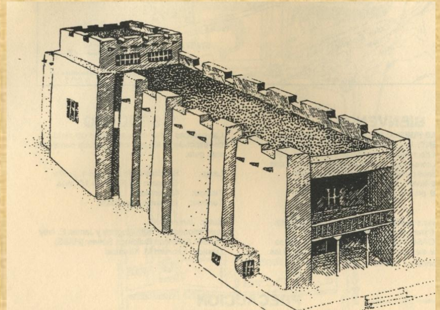
Dibujo de la Misión de San Gregorio de Abó completa.
